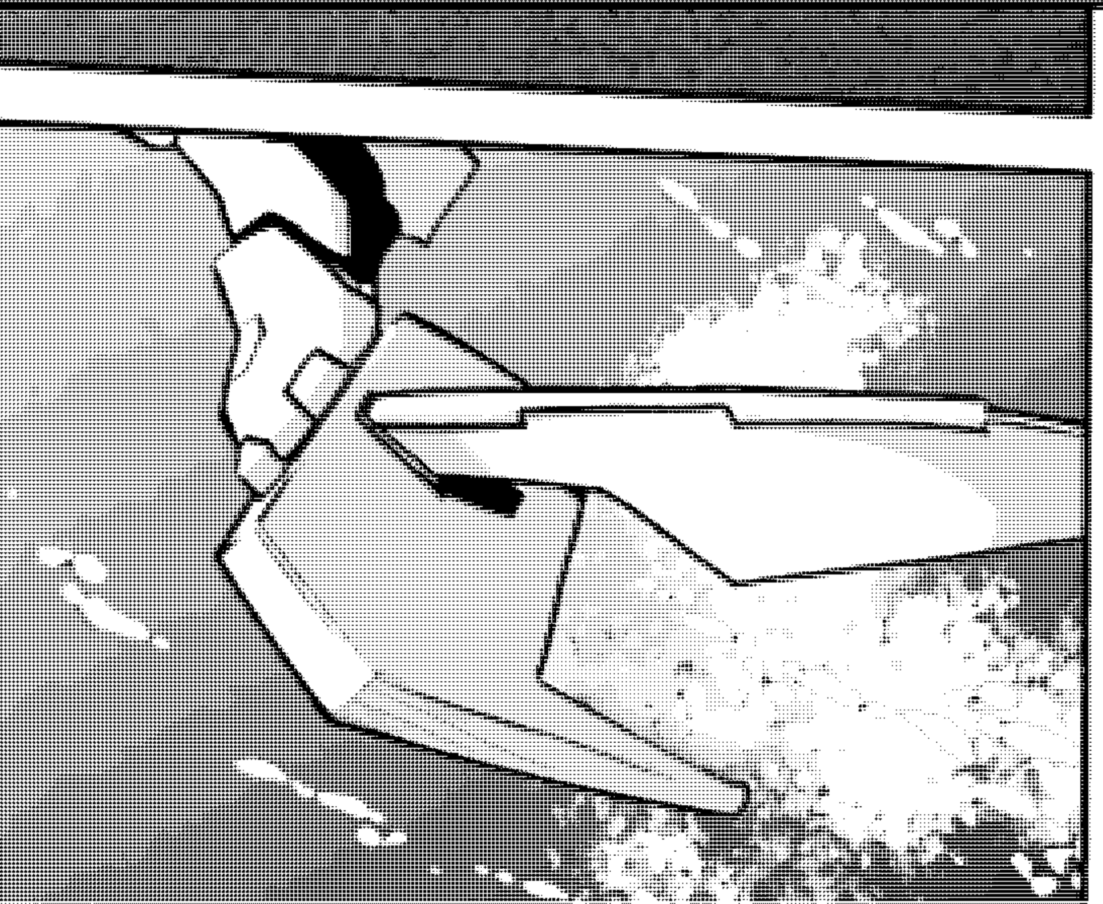
海形海山 深度2500 牙汐号
